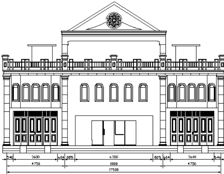
Eerste concept plan van het kantoor met aan weerszijden een huis voor de staf van Spie-en.
